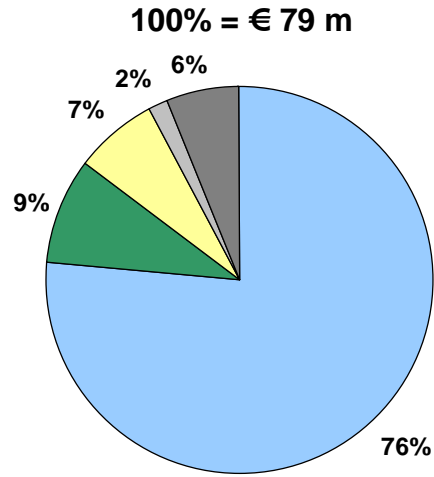
EBIT
