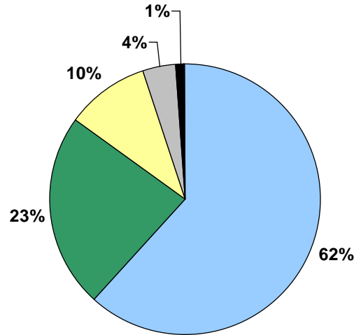
EBIT
